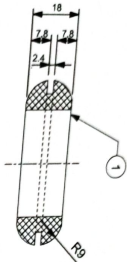
SEC.-A-A
