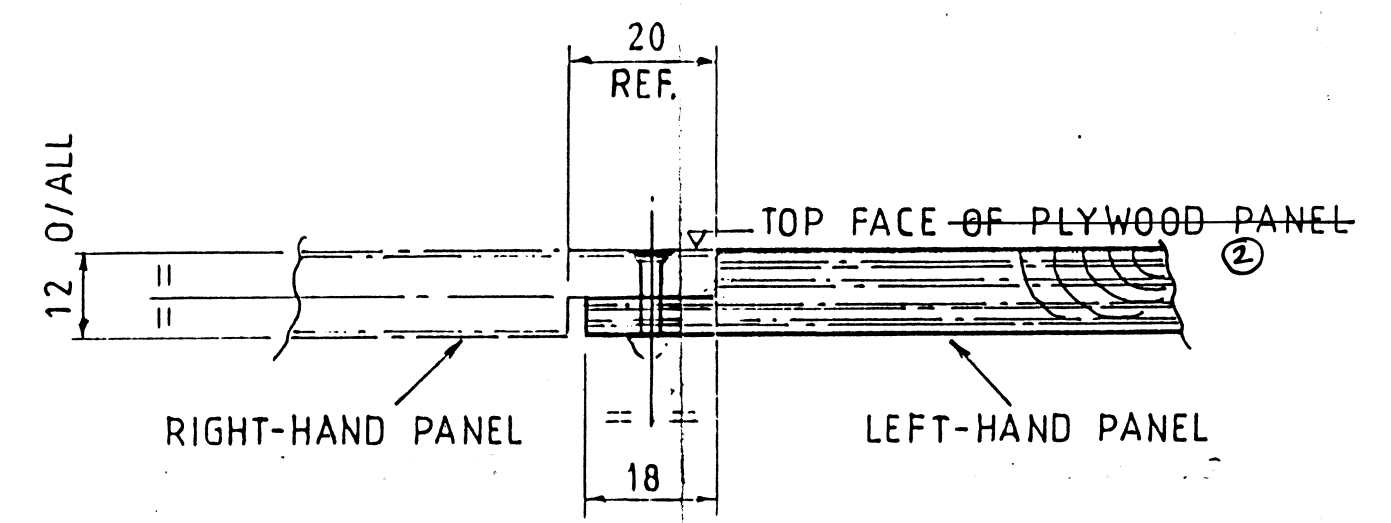
SECTION A-A (JOINT) SCALE 1:1
